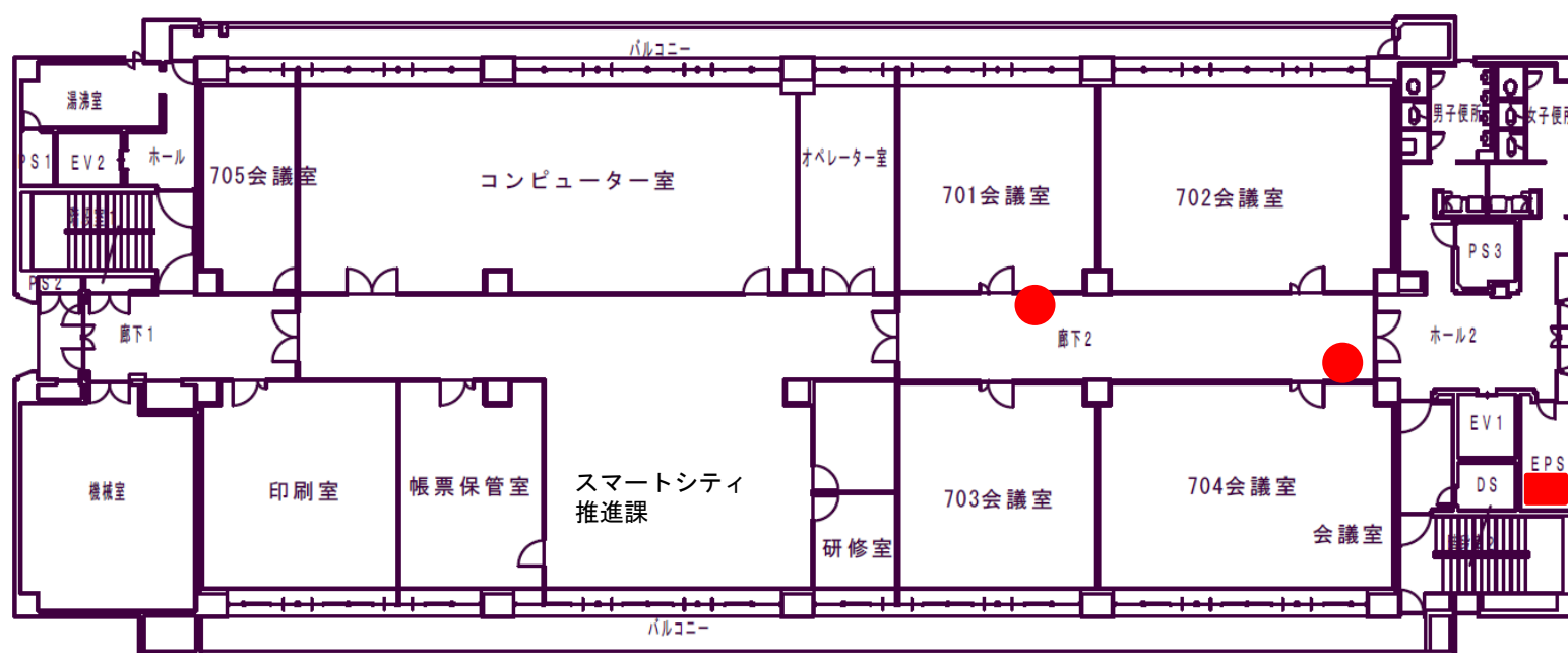
7階平面図 1:200
