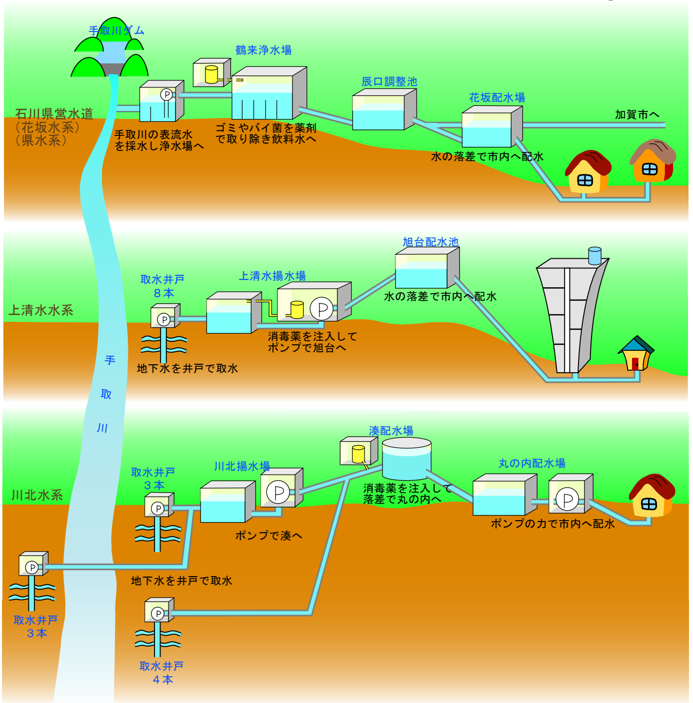
図2 配水フロー
