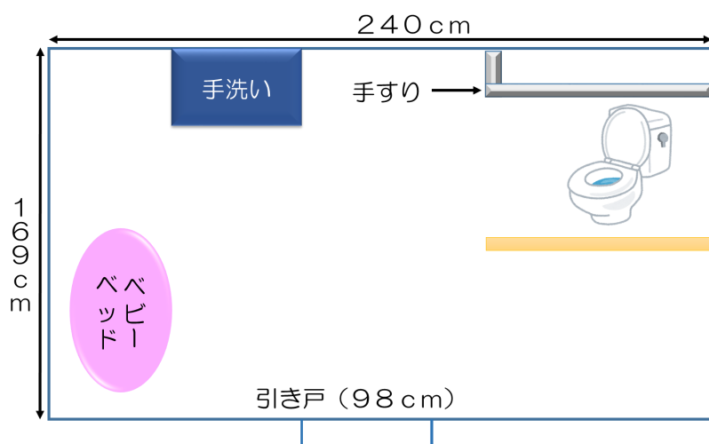
多目的トイレのレイアウト
