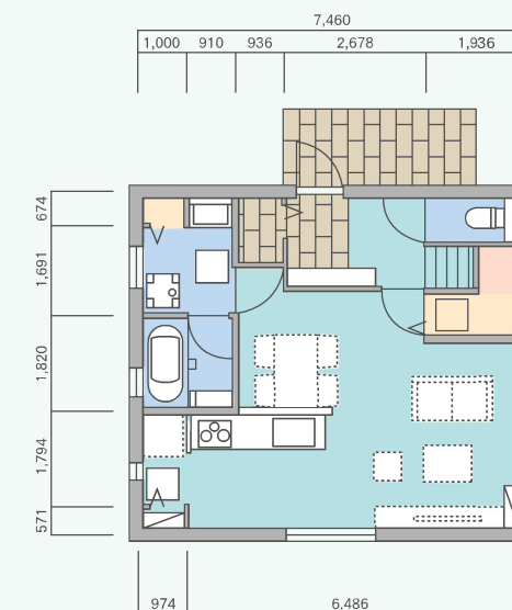
1階平面図
