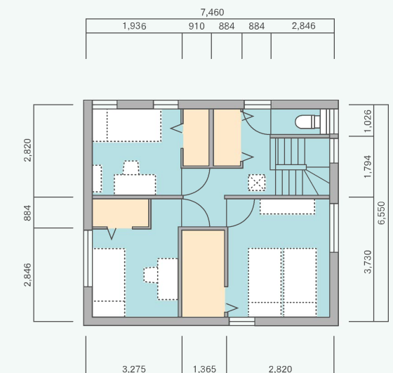
2階平面図
