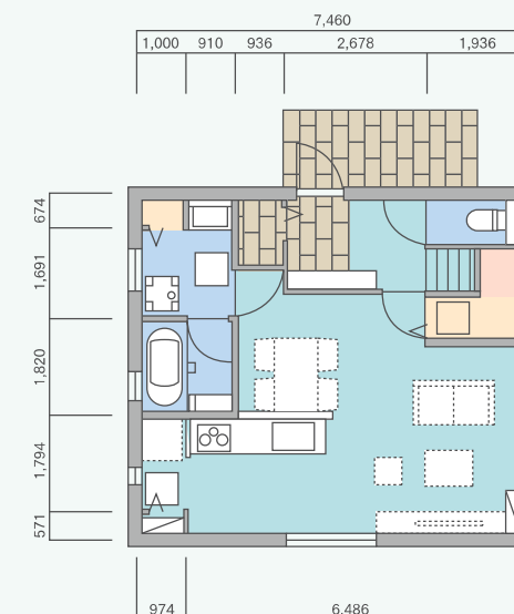
1階平面図
