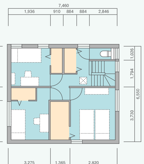
2階平面図
