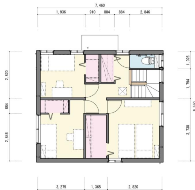
2階平面図
