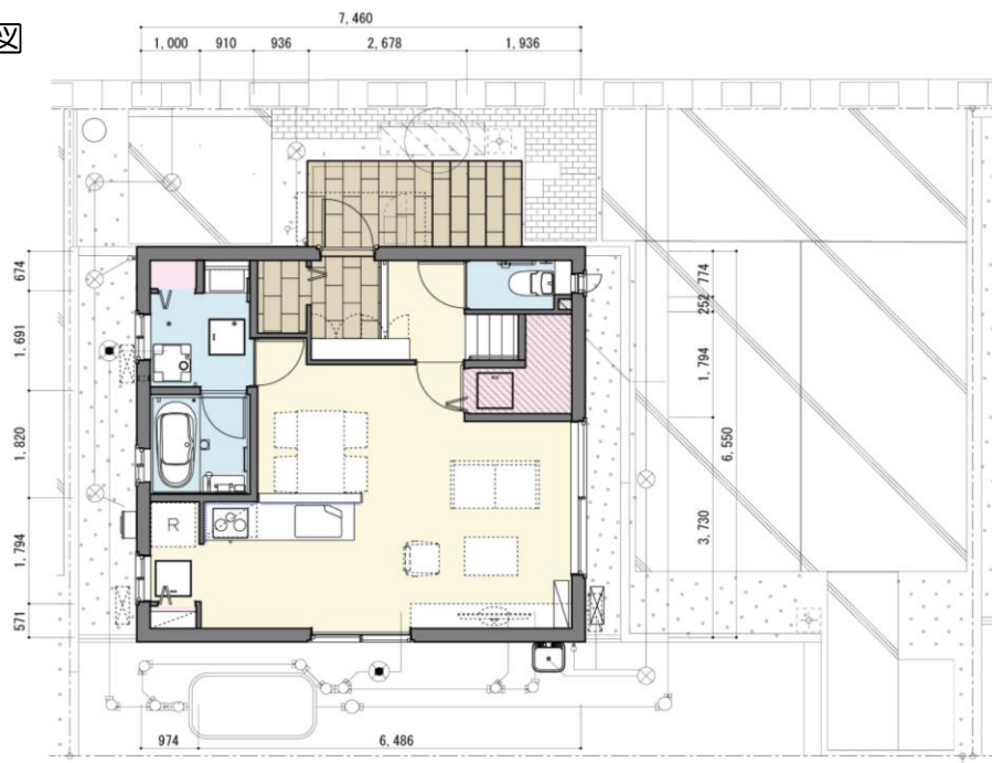
1階平面図
