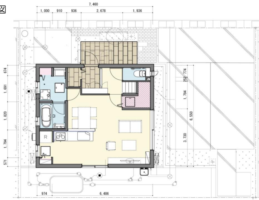
1階平面図
