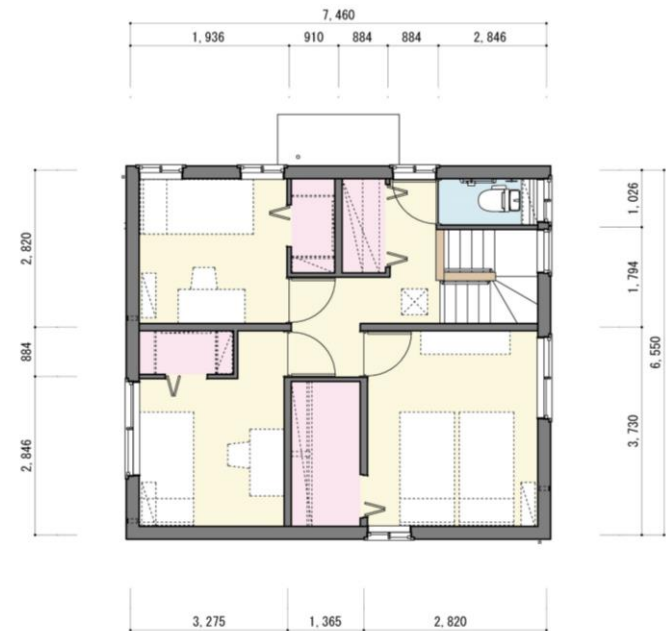
2階平面図
