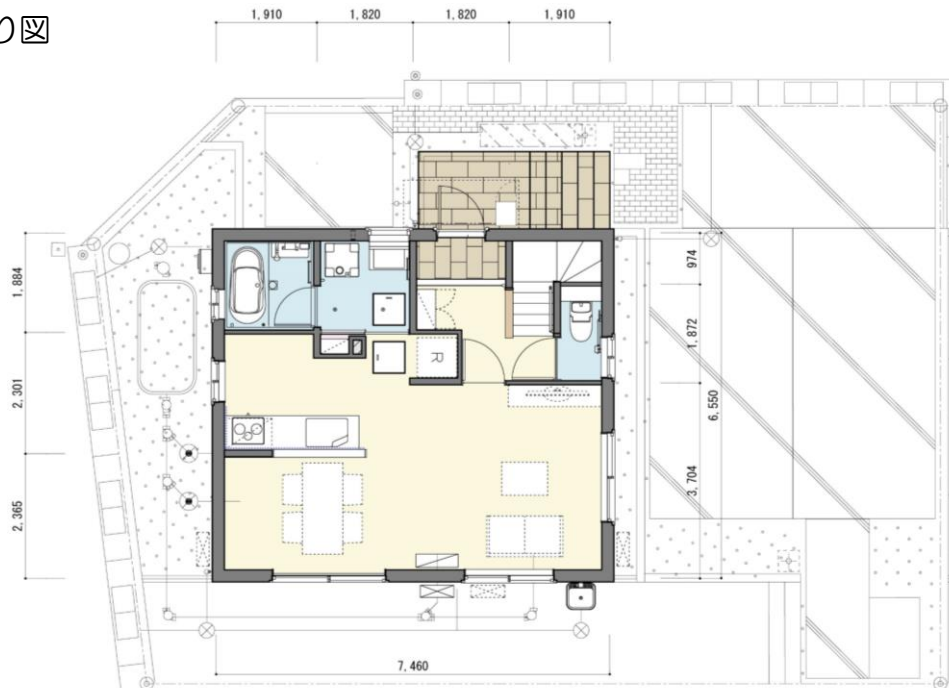
1階平面図
