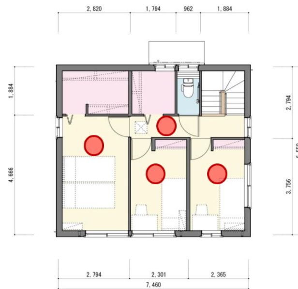
2階平面図
