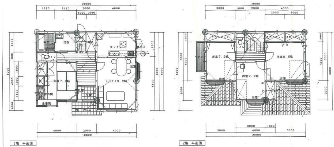
間取り図
