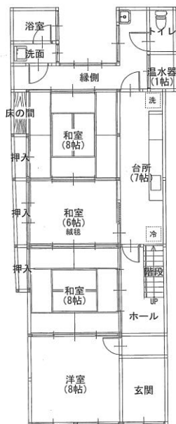
1階 平面図
