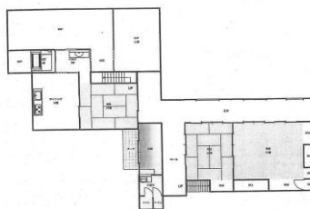
1階 縮尺 1/150
