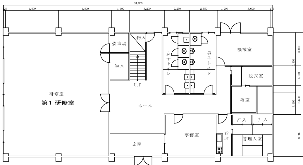
1 F 平面図 S=1/100
