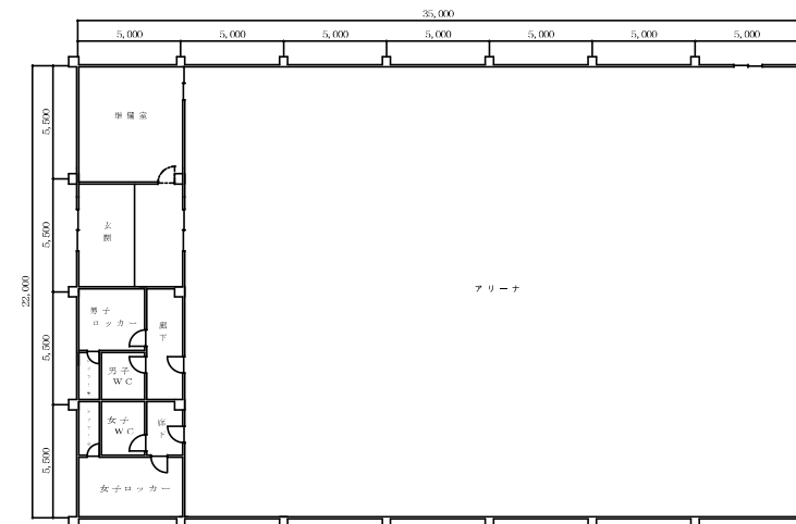
1 F 平面図 S=1/300
