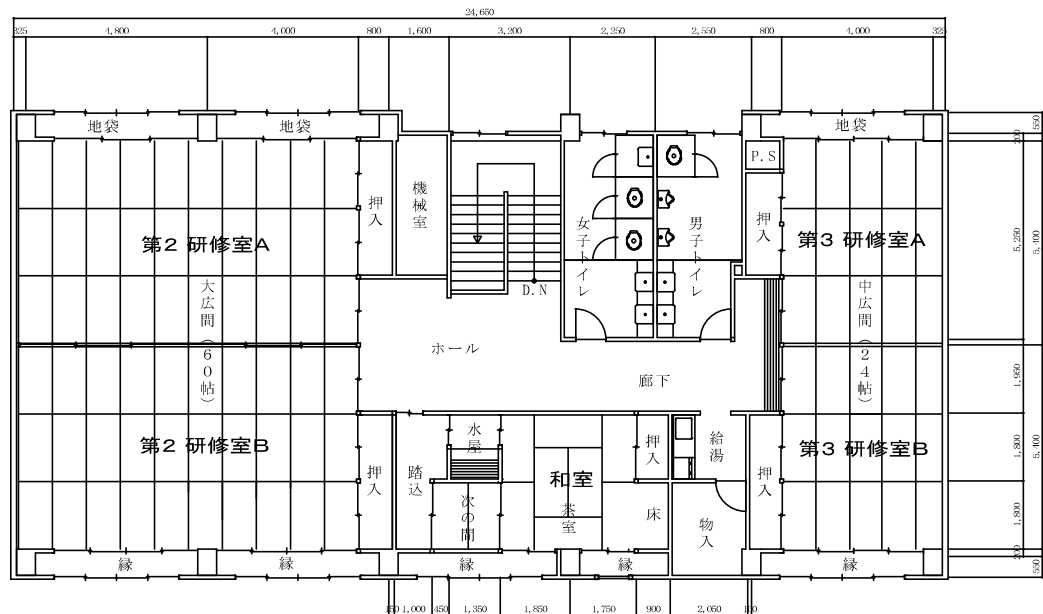
2 F 平面図 S=1/100
